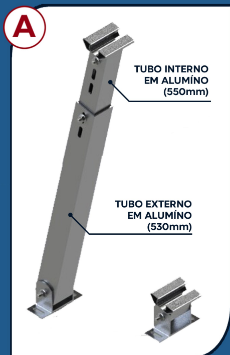
TRF001 SUPORTE METÁLICO ALUMÍNIO VERTICAL - CORREÇÃO DE INCLINAÇÃO 5 UNIDADES
